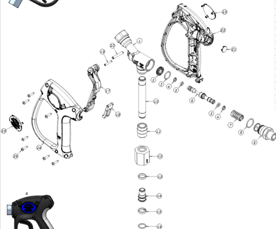
DETTAGLIO B
